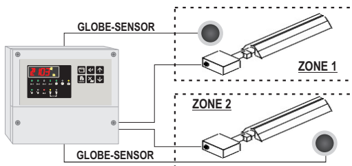
MODO 7: 2 ZONE TERMICHE - 1+1 BRUCIATORI BISTADIO MODE 7: 2 THERMAL ZONES - 1+1 TWO FLAME BURNERS
