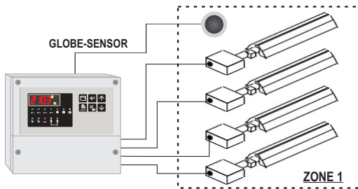
MODO 1: 1 ZONA TERMICA - 4 BRUCIATORI MONOSTADIO MODE 1: 1 THERMAL ZONE - 4 SINGLE FLAME BURNERS
