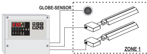
MODO 5: 1 ZONA TERMICA - 2 BRUCIATORI BISTADIO MODE 5: 1 THERMAL ZONE - 2 TWO-FLAME BURNERS
