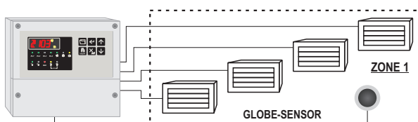
MODO 9: 1 ZONA TERMICA - 4 GENERATORI D'ARIA CALDA MODE 9: 1 THERMAL ZONE - 4 WARM AIR GENERATORS
